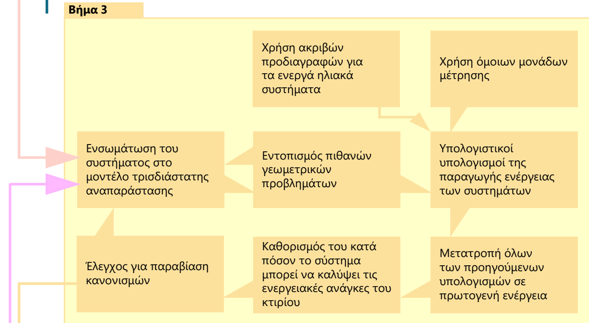
Εικόνα 21 Η βασική μεθοδολογία για το τρίτο βήμα, που ασχολείται με την ενσωμάτωση ενός επιλεγθέντος ενεργητικού ηλιακού συστήματος και την προσομοίωση της ενεργειακής παραγωγής του.
