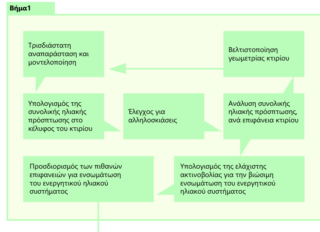
Εικόνα 19 Η βασική μεθοδολογία για το πρώτο βήμα, που ασχολείται με την παθητική ενεργειακή ανάλυση του κτιρίου ή της ομάδας κτιρίων, σε αστικό επίπεδο.
