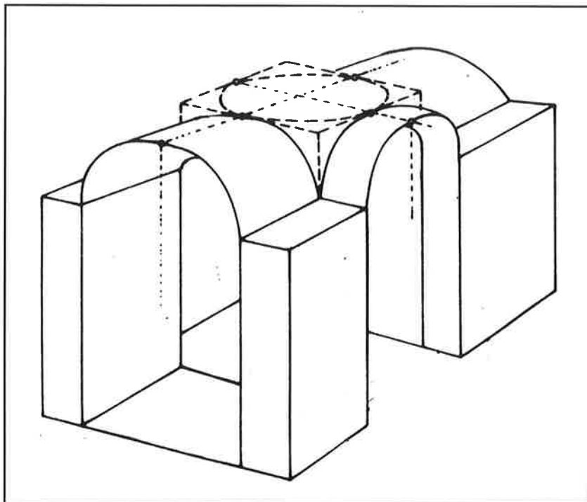
Σχέδ. 5 Σχέδιο που δείχνει τον αναλογικό τρόπο στέγασης του κεντρικού χώρου της αίθουσας 1. (Ν. Μουτσόπουλος, Εκκλησίες της Καστοριάς).
